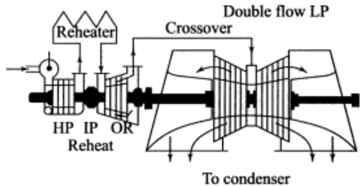
(D) Single reheat cycle
