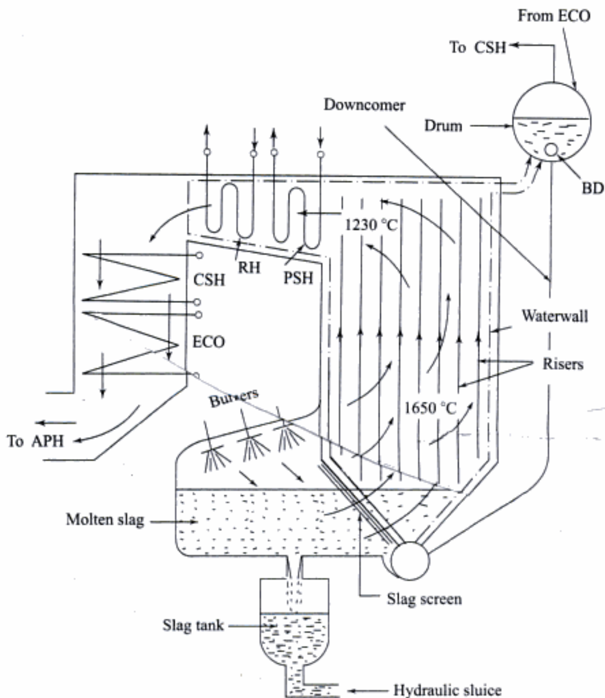
Fig. 5.24 Wet-bottom furnace
