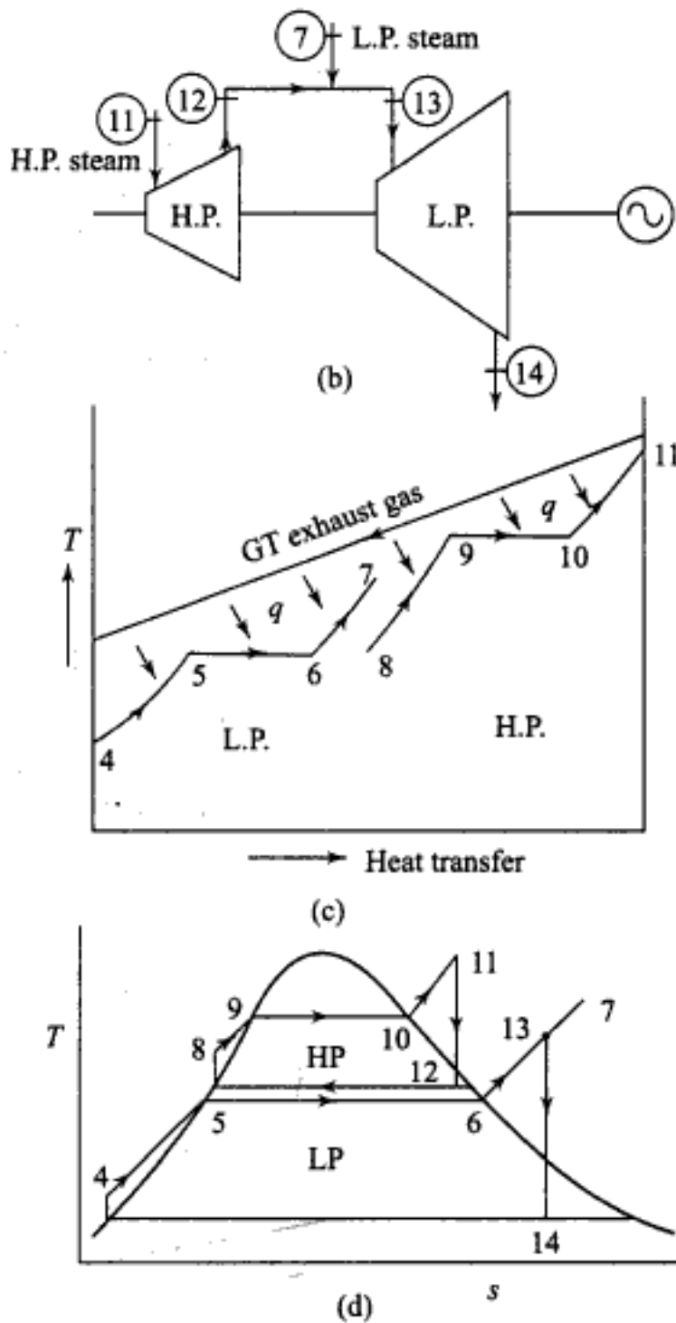
Fig. 3.13 Dual pressure steam cycle (a) HRSG, (b) H.P. and L.P. turbines, (c) T-q diagram, (d) T-s diagram
