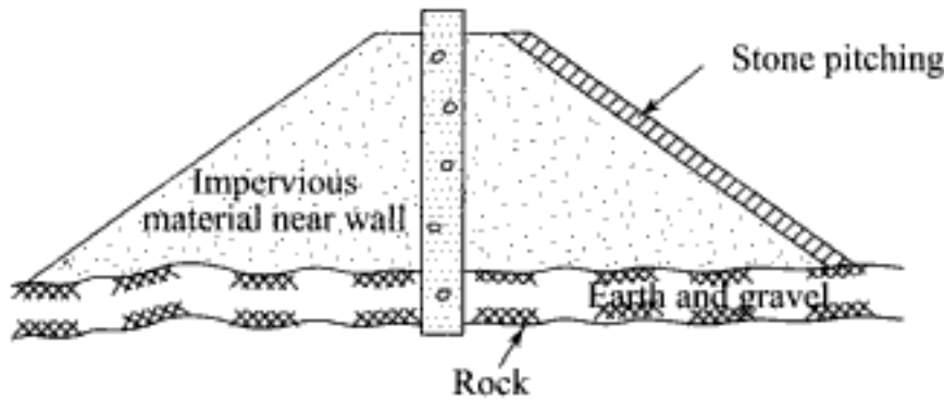
Fig. 10.11 Earth dam
